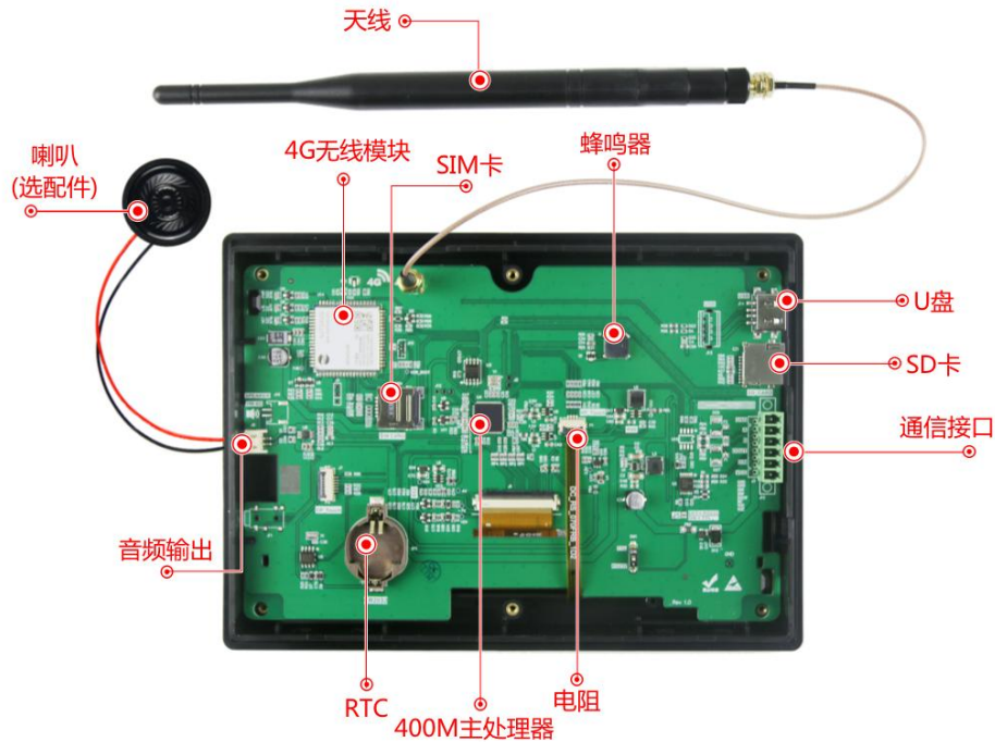
图 1-2 硬件配置图
