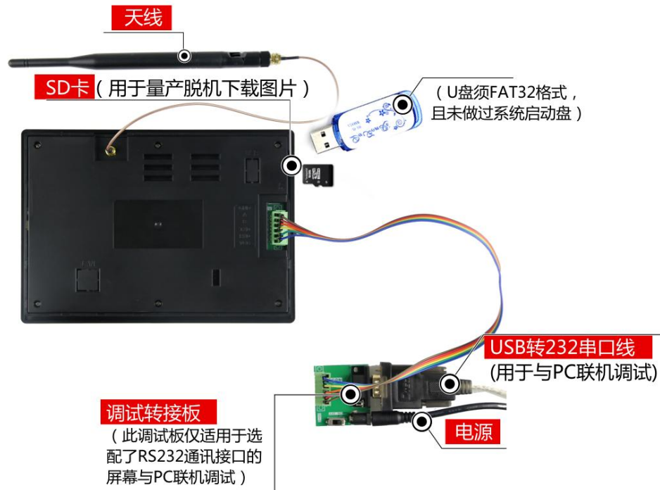
图 1-3 RS232 调试工具图
