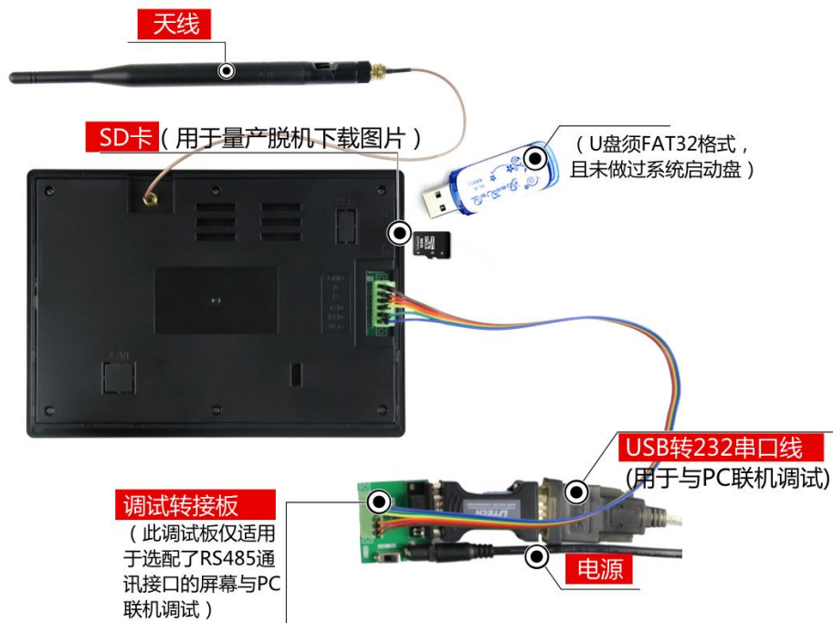
图 1-4 RS485 调试工具图
