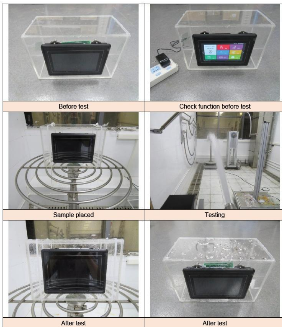
图 6-5 防水测试图
